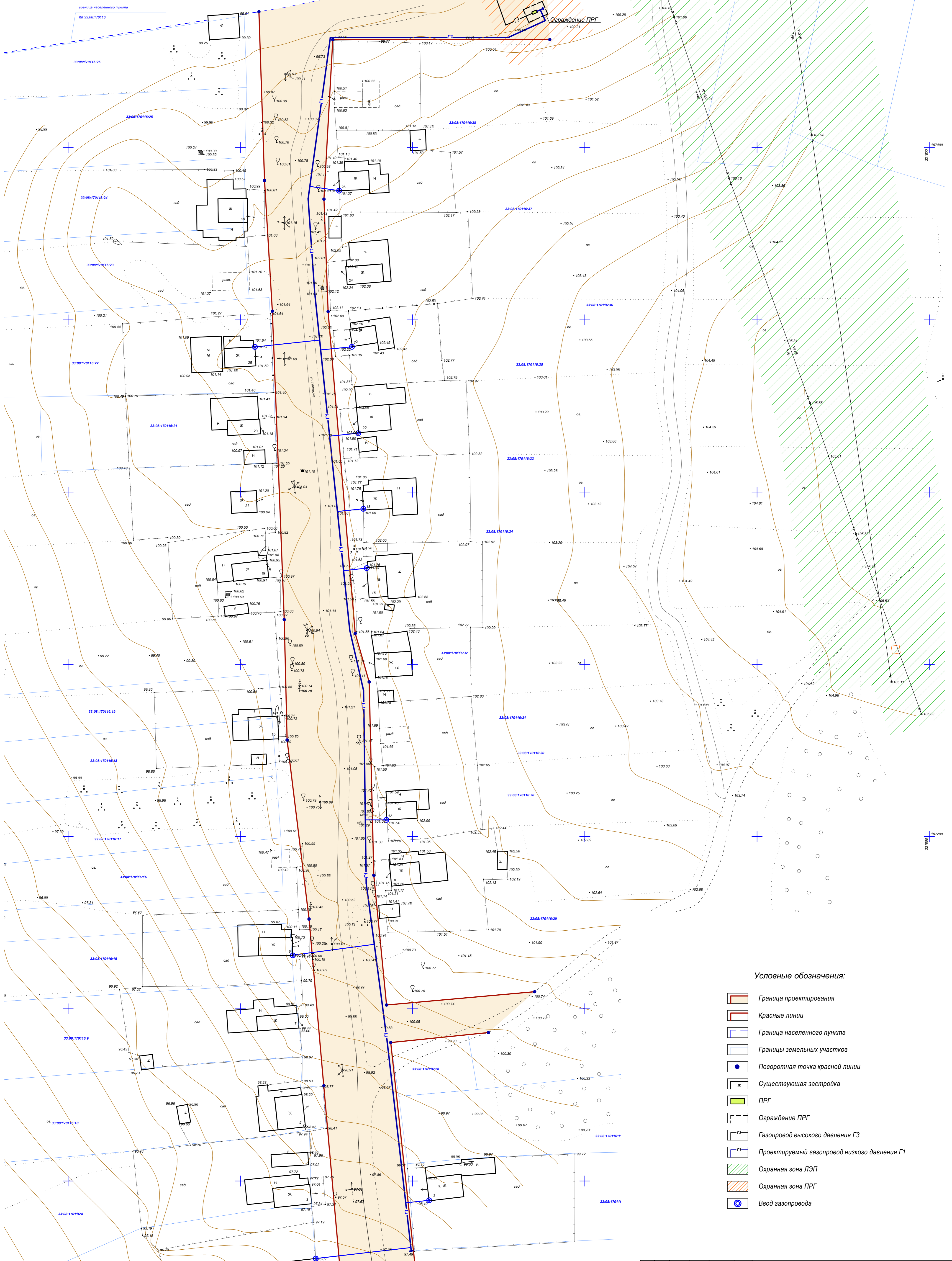
Схема 3. План газопровода М 1:500 (Основной чертеж)
