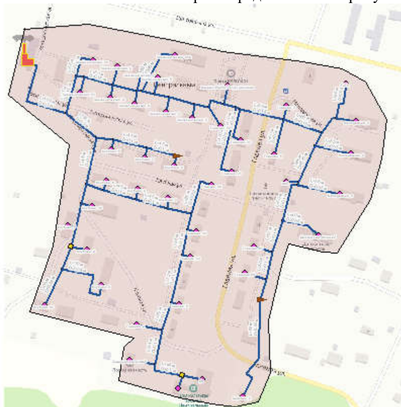
Рисунок 2 - Зона действия источника тепловой энергии (Котельная п. Центральный)
