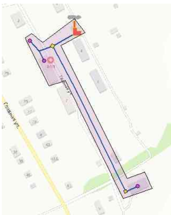
Рисунок 3 - Зона действия источника тепловой энергии (Котельная д. Воробьевка)
